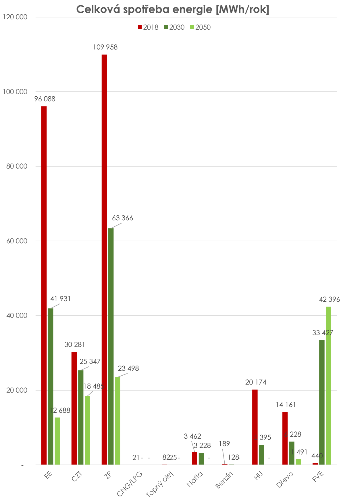
Obrázek 30: Graf – Celková spotřeba energie dle energonositele [MWh/rok]
