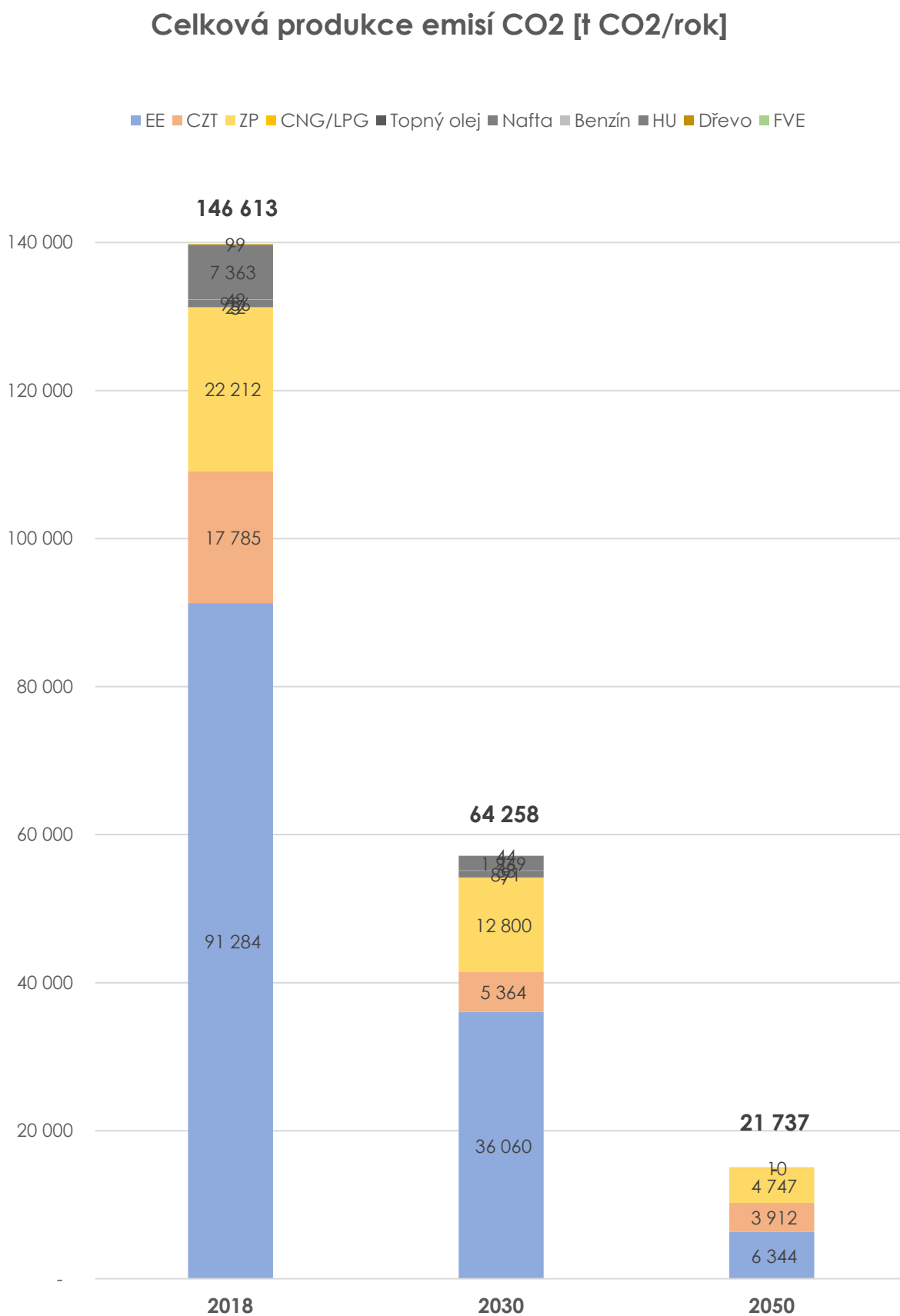
Obrázek 34: Graf - Celková produkce emisí CO 2 [t CO 2 /rok]
