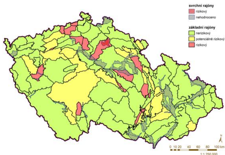
Obrázek 8 - Hydrogeologické rajony potenciálně zranitelné vůči nedostatku vody, zdroj: VÚV
