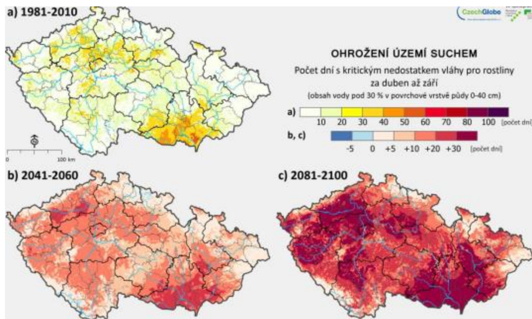
Obrázek 9 - Výhled možného následku změny klimatu pro vláhový deficit půdy v porovnání v současnosti a výhledech pro rok 2050 a 2100 při zachování současného trendu změny klimatu podle průměrného scénáře vývoje. Zdroj: CzechGlobe, MENDELU
