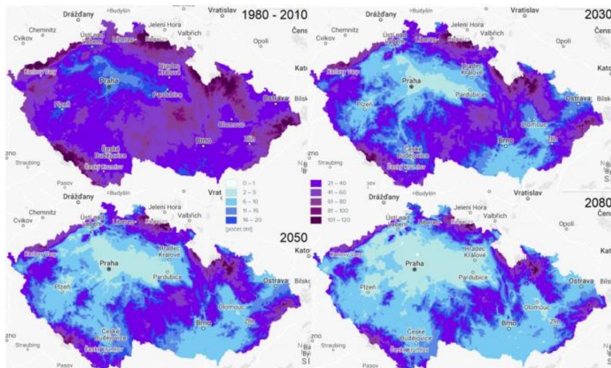
Obrázek 10 - Budoucí vývoj počtu dní s pokrývkou nad 10 cm pro střední emisní scénář (klimatickazmena.cz)
