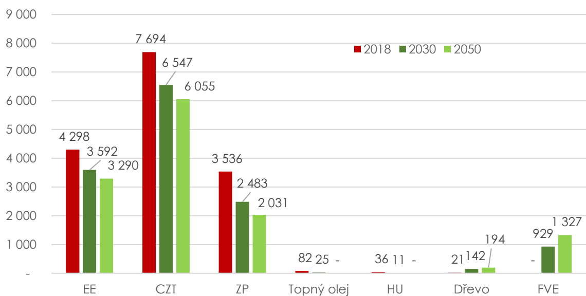
Obrázek 5: Graf – vývoj spotřeby energií v sektoru budov obcí [MWh/rok]
