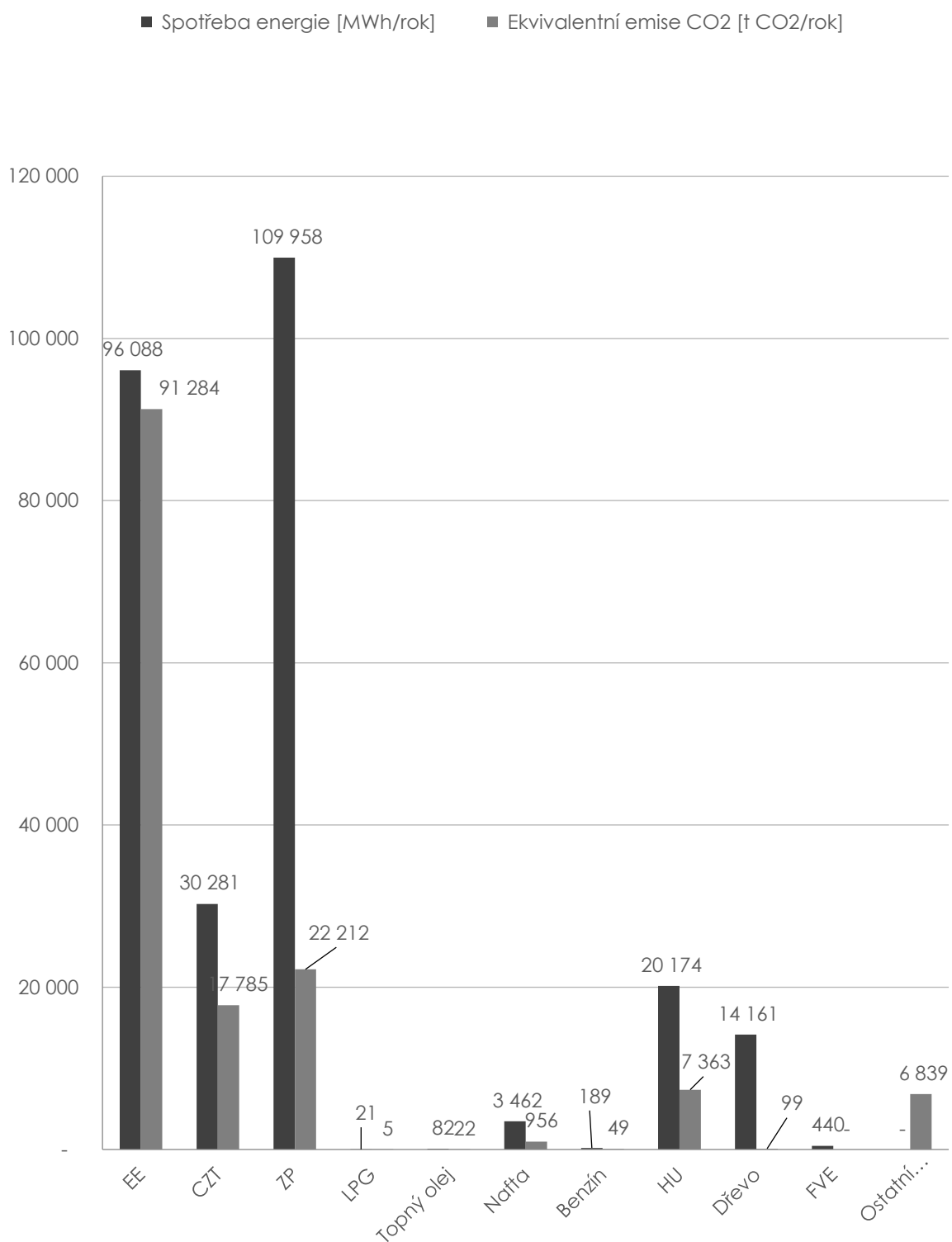
Obrázek 2: Celková spotřeba energie a ekvivalentní emise CO 2 dle energonositelů za rok 2018
